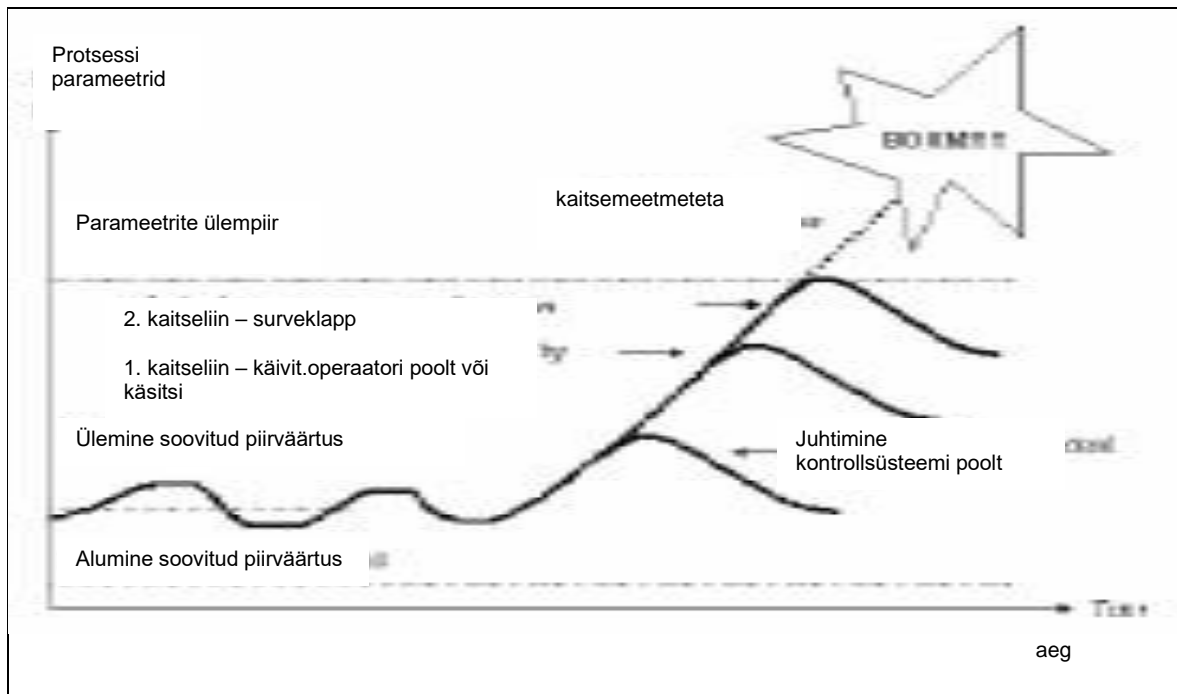
Joonis 1.1 Juhtimis- ja ohutussüsteemi funktsioon protsessi parameetri jaoks
